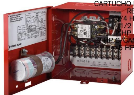
CAJA DE CONTROL PARA 1/3, 3/4 1 1/2 Y 2 HP COD.880-041-5
